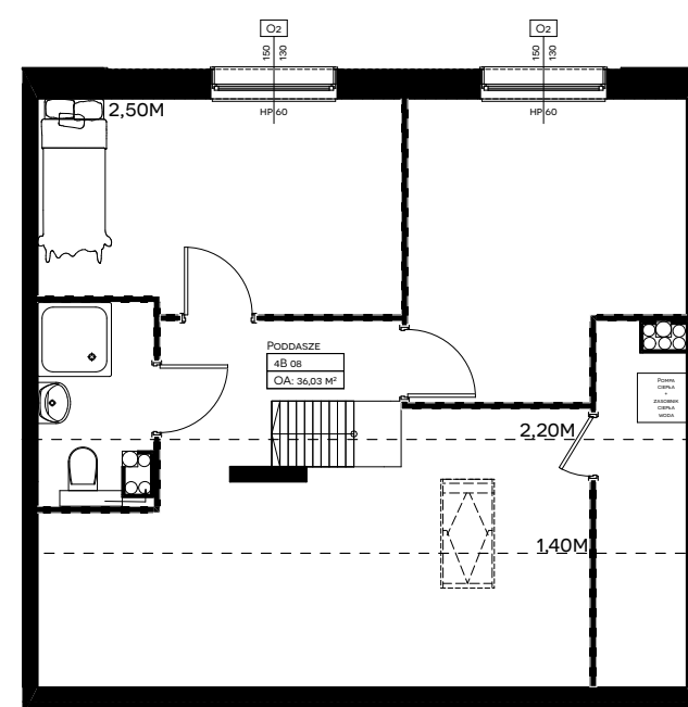
PODDASZE
